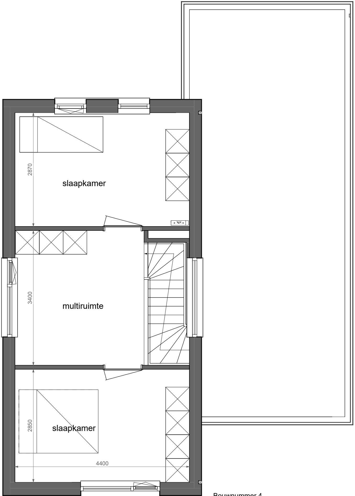
Bouwnummer 4 Bungalow met opbouw Eerste verdieping Schaal 1:50
